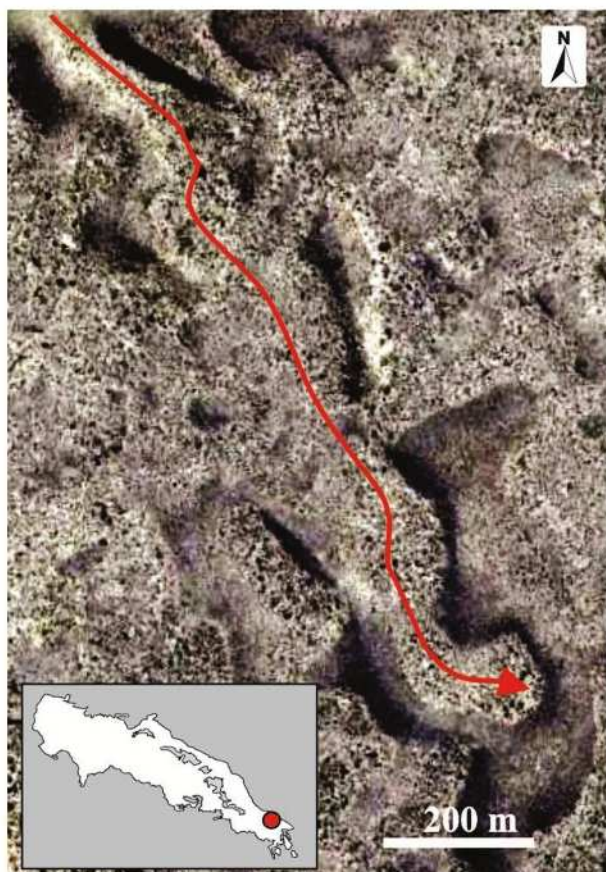
Figura 4. Estructura de un flujo de lava interpretada como un remanente de un túnel de lava con el techo derrumbado.
