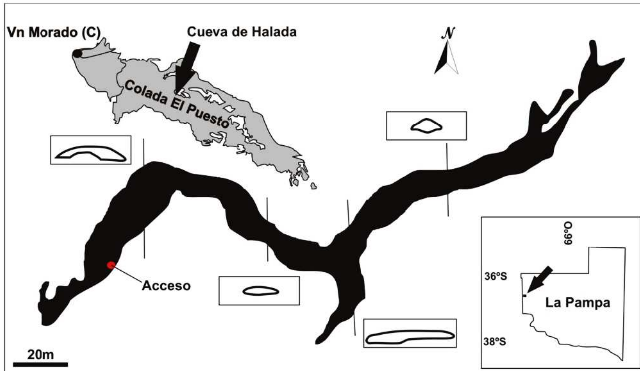
Figura 2. Cueva de Halada. Ubicada en el flujo de lava de El Puesto. Datos de morfología del plano tomados de Bertotto (1996) y Martínez (1998). Los recuadros indican las secciones transversales estudiadas en algunos sectores del túnel principal (Martínez, 1998). Obsérvese la asimetría de la sección en los segmentos cercanos a las curvas.
