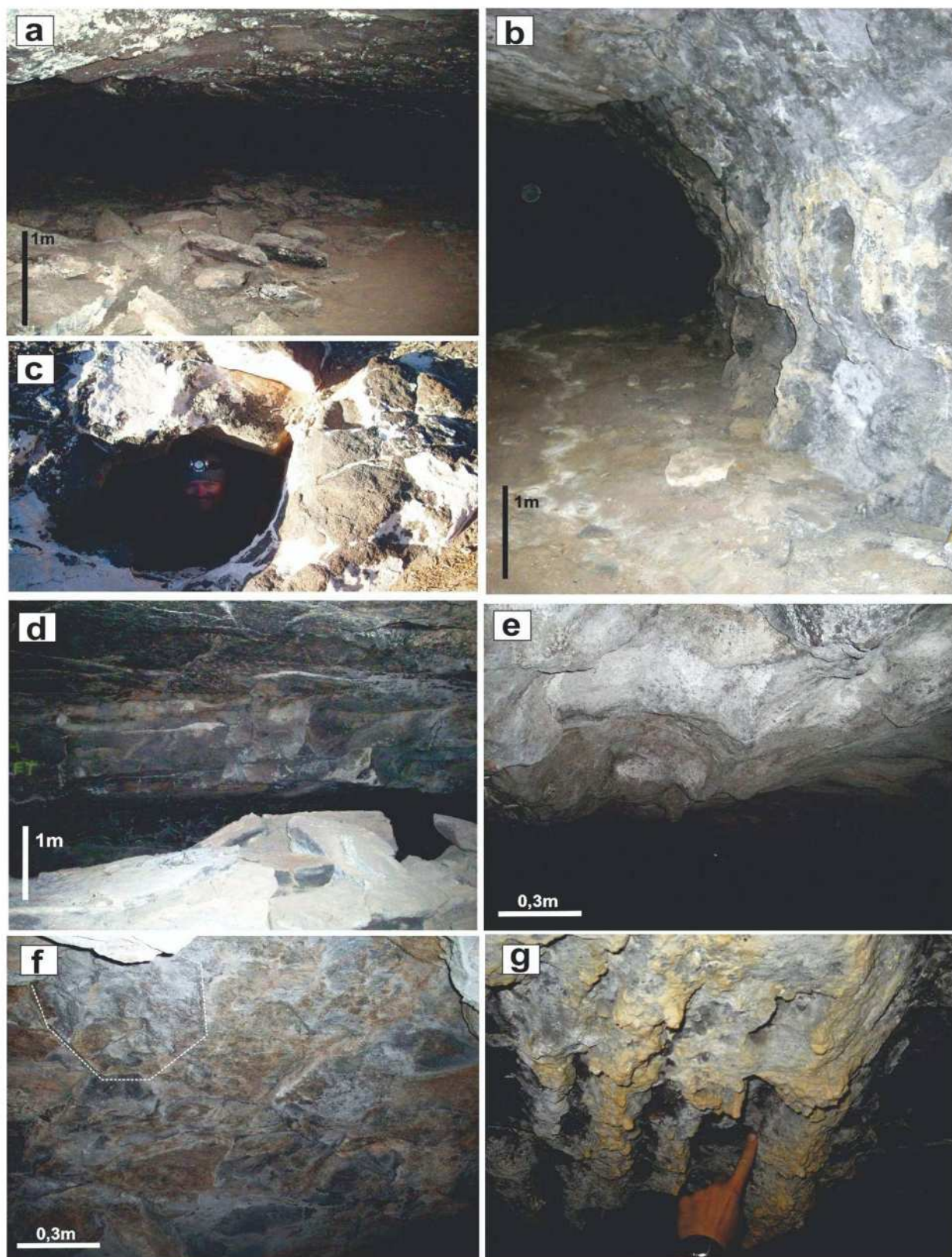
Figura 3. Cueva de Halada. Estructura interna. a y b) Sección transversal del túnel bajo la entrada de acceso. Esta sección es la más ancha de toda la estructura y corresponde al pasaje principal. Presenta un techo abovedado y una altura máxima de 2 m; c) Entrada de acceso al túnel; d) Estructura de las paredes y el techo, y rocas desprendidas del techo; e) Techo con una estructura ondulada tipo "caja de
