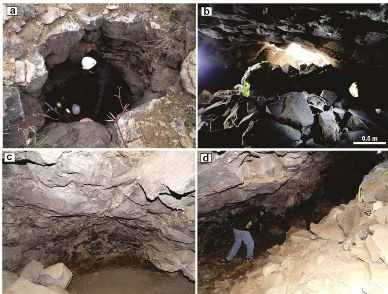
Figura 7. Cueva El Julepe. Imágenes. a) Entrada desde la superficie. b) Acceso, ubicado a unos dos metros de la superficie. En primer plano, se observan rocas desprendidas del techo de la cueva. c) Presencia de carbonatos y sulfatos que cubren las paredes y el techo de la cueva y rellenan las fracturas. d) Sector central con rocas desprendidas del techo de la cueva y bordes internos de la cueva prácticamente sin bloques desprendidos.
