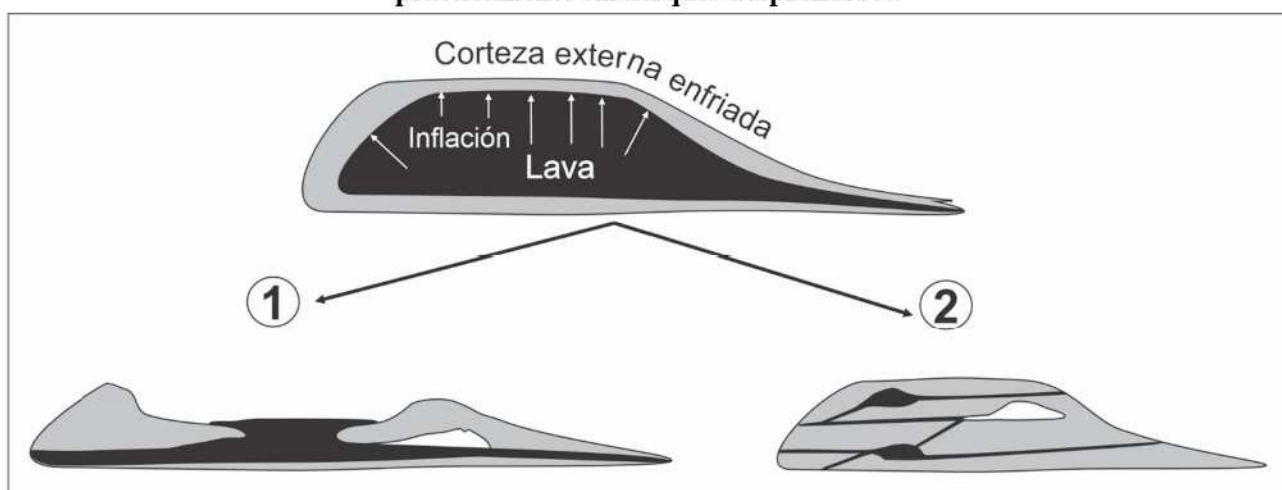
Figura 8. Representación esquemática del origen inferido de la cueva El Julepe. Inicialmente, el levantamiento de techo plano se produjo por inflación, como resultado de la inyección de lava bajo la corteza superficial enfriada. En el caso 1, la lava se drena hacia la superficie o internamente a través de un túnel de lava más grande (ej. cueva de Halada), provocando el colapso del techo del
