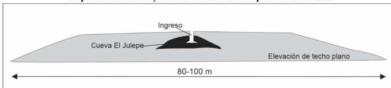
Figura 5. Diagrama de la cueva El Julepe. a) Sección transversal de la cueva. Se observa un techo severamente fracturado y un suelo cubierto por desprendimientos de rocas, principalmente en la sección central de la cueva. Hacia los márgenes interiores de la cavidad, la presencia de bloques desprendidos disminuye. También se muestra el plano de la cavidad.
