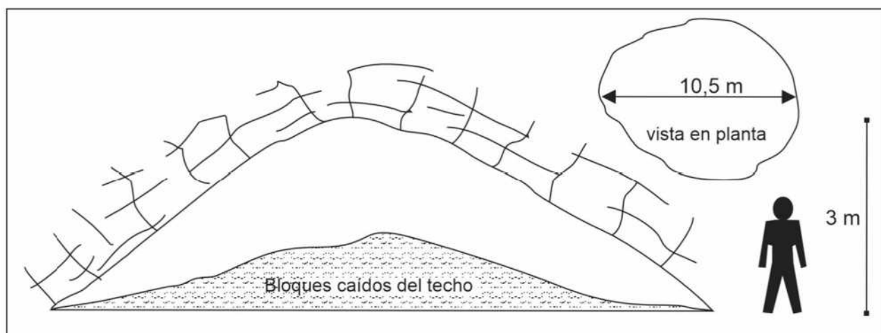
Figura 5. Diagrama de la cueva El Julepe. a) Sección transversal de la cueva. Se observa un techo severamente fracturado y un suelo cubierto por desprendimientos de rocas, principalmente en la sección central de la cueva. Hacia los márgenes interiores de la cavidad, la presencia de bloques desprendidos disminuye. También se muestra el plano de la cavidad.
