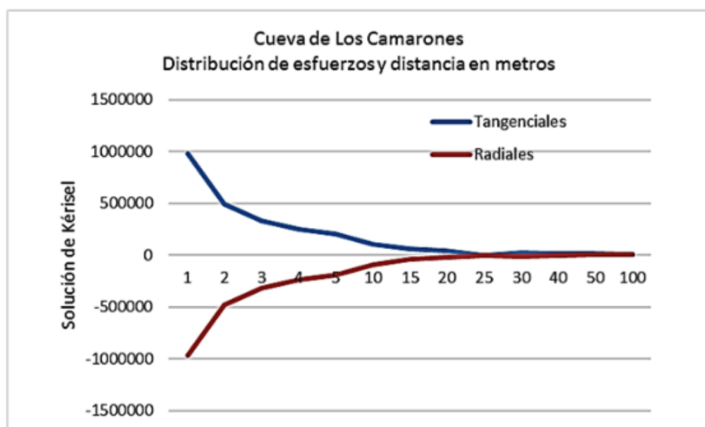
Fig. 5. Solución del campo de esfuerzos horizontales para el campo de esfuerzos en la Cueva de Los Camarones (Molerio, 2017) según el Modelo de Kérisel.
