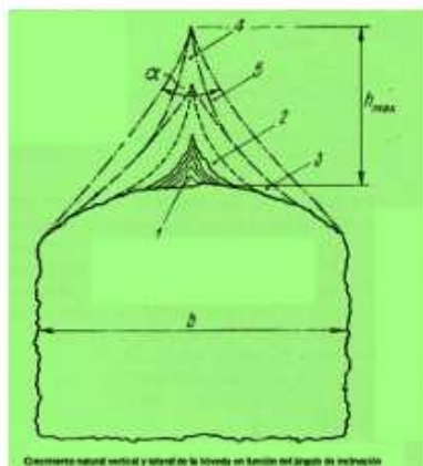
Fig. 10. Crecimiento natural vertical de la bóveda en función del ángulo del arranque (Széchy, 1967)
