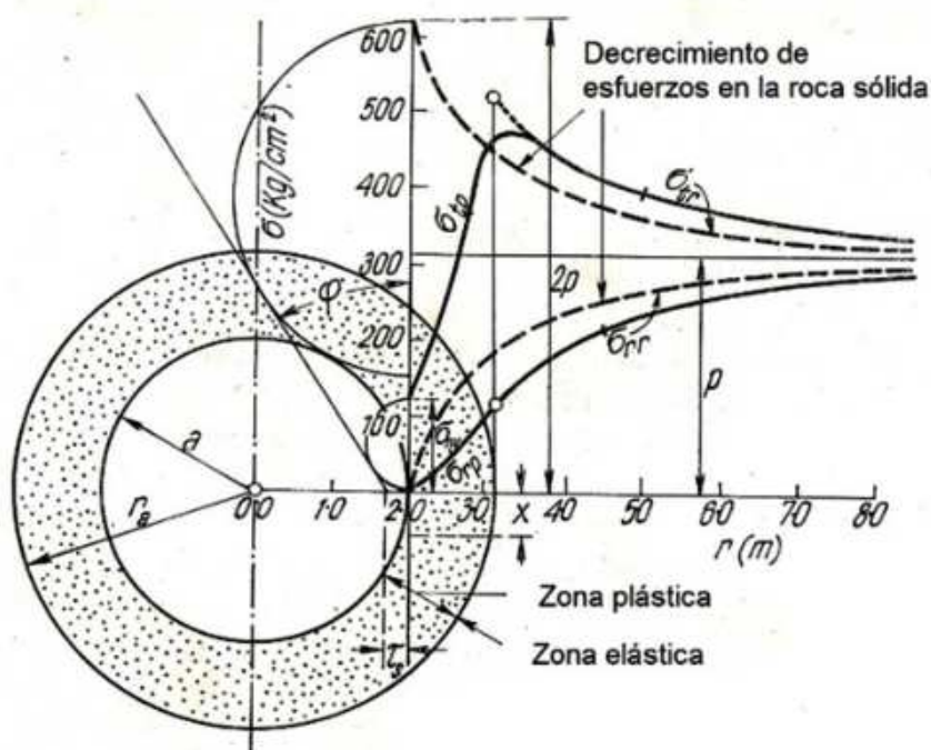
Desarrollo de esfuerzos radiales y tangenciales en una cavidad circular excavada en rocas elásticas y plásticas (Kastner)
