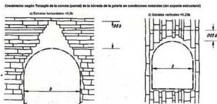
Fig. 9. Crecimientos teóricos de la clave de las bóvedas (según Terzaghi) en relación con la estratificación y el ancho de la sección de la galería
