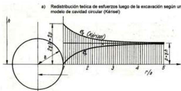
Fig. 4. Solución de Kérisel para la distribución de esfuerzos tangenciales y radiales en una cavidad circular (tomado de Széchy, 1967). Nótese que, en el perímetro, el esfuerzo tangencial se duplica mientras que el radial se hace cero
