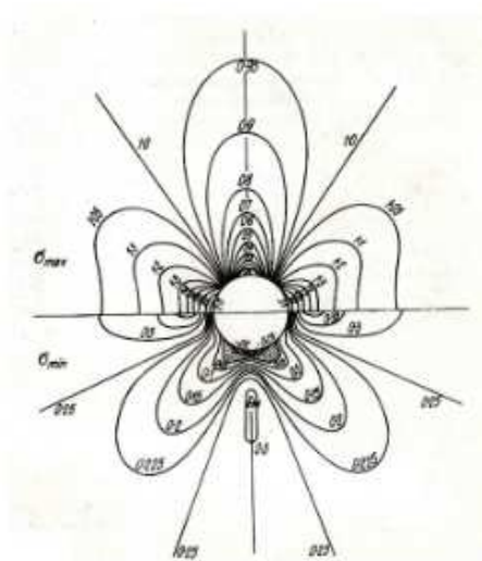
Fig. 8. Isobaras de tensiones en una cavidad circular (Széchy, 1967)
