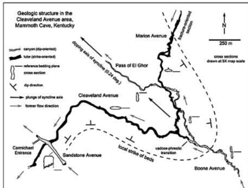
Fig. 11. Ejemplo del control estructural sobre la orientación de galerías de Cleveland avenue en Mammoth Cave (tomado de Palmer, 2016).
