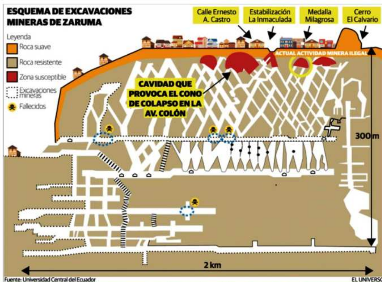
Fig. 1. Esquema de distribución en perfil de galerías mineras en el casco urbano patrimonial de la Ciudad de Zaruma, El Oro, Ecuador. (Fuente Universidad Central del Ecuador. Tomado del Diario el Universo). Obsérvese la proximidad de galerías de diferente sección, orientación, longitud, accesos, cercanía a la superficie y también reforzamientos deficientes.
